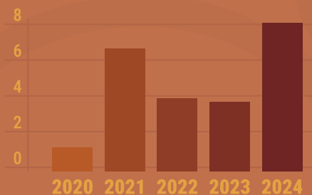
CROISSANCE PIB
