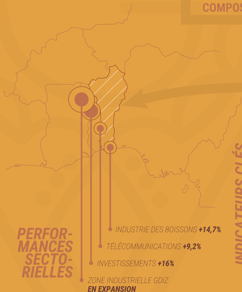
CROISSANCE PIB
